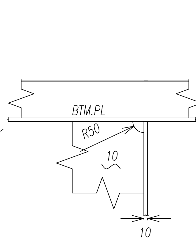
DTL. C
