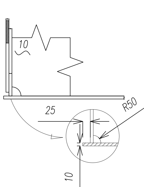
DTL. B
