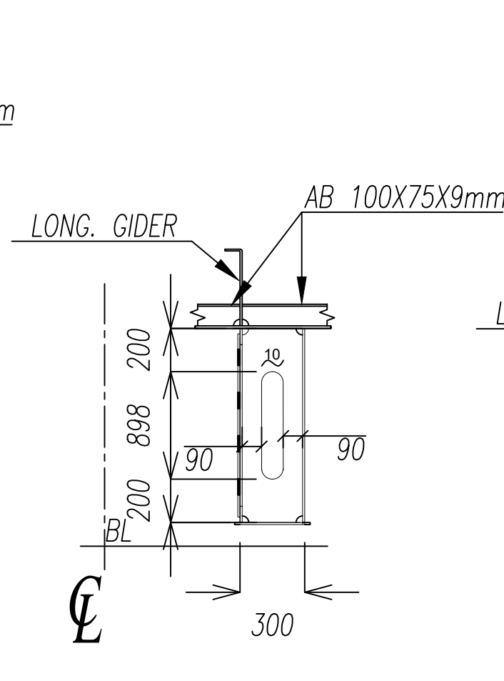
FRAME 1 +762
