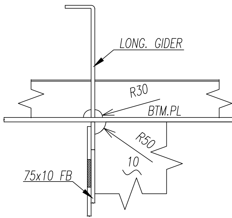
DTL. A
