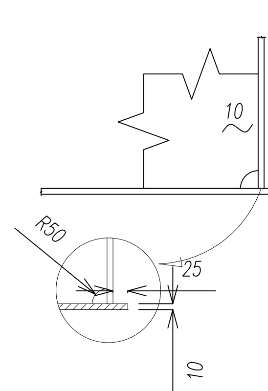
DTL. D
