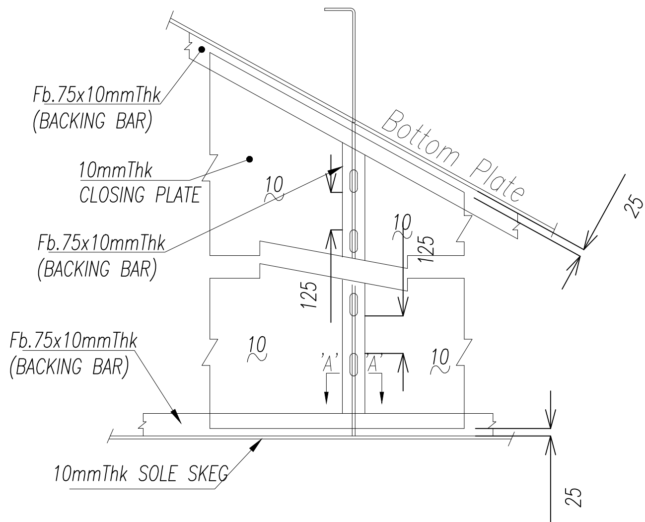
SLOT WELD DTL 1:2
